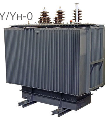
ТМГ 21 производства МЭТЗ им. В.И. Козлова
