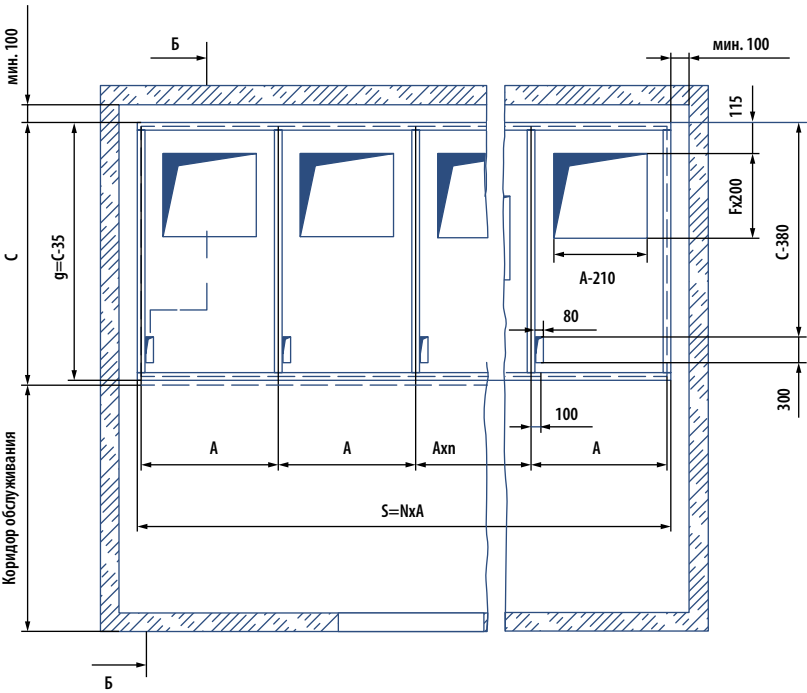
Рис. 39. Пример конструкции фундаментной рамы (вид сверху)
