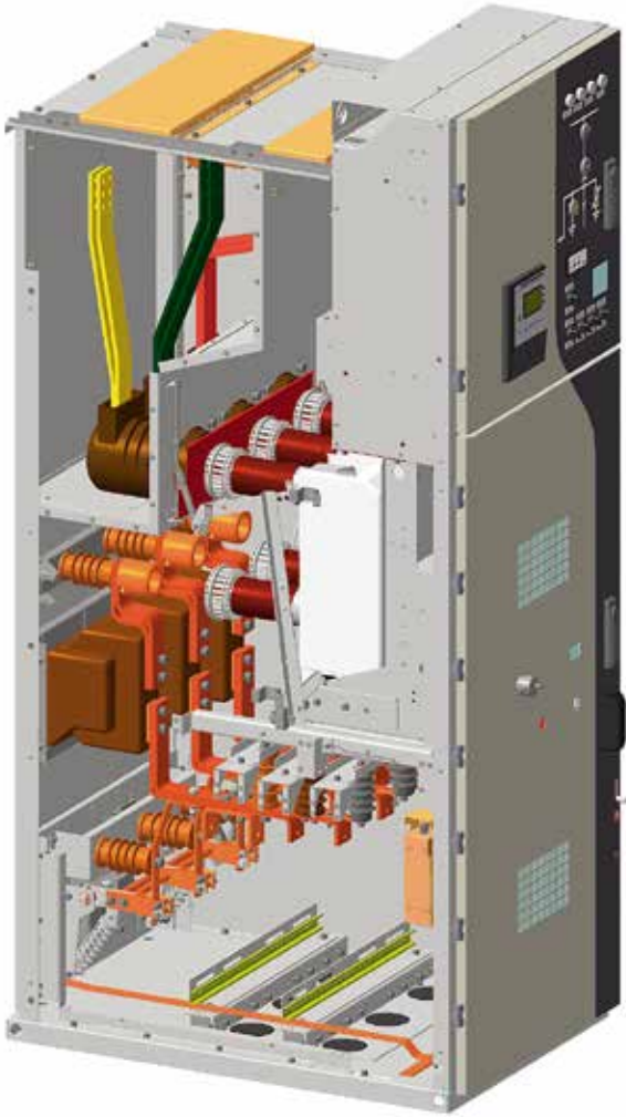
Рис. 3. КРУ «Элтима Лайт». Общий вид
