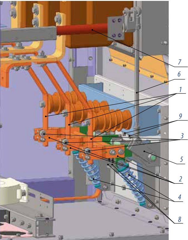
Рис. 23. Заземлитель с ручным управлением
