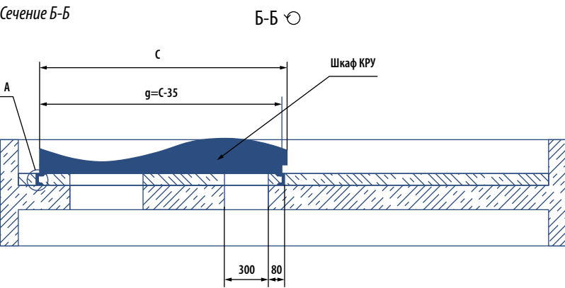
Рис. 40. Пример конструкции фундаментной рамы (разрезы)
