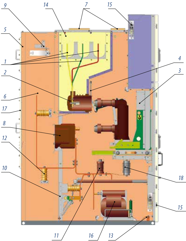
Рис. 4. Пример шкафа с силовым выключателем и ТН. Кабельный ввод сзади
