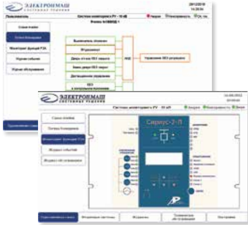
Рис. 35. Экраны системы мониторинга и управления КРУ
