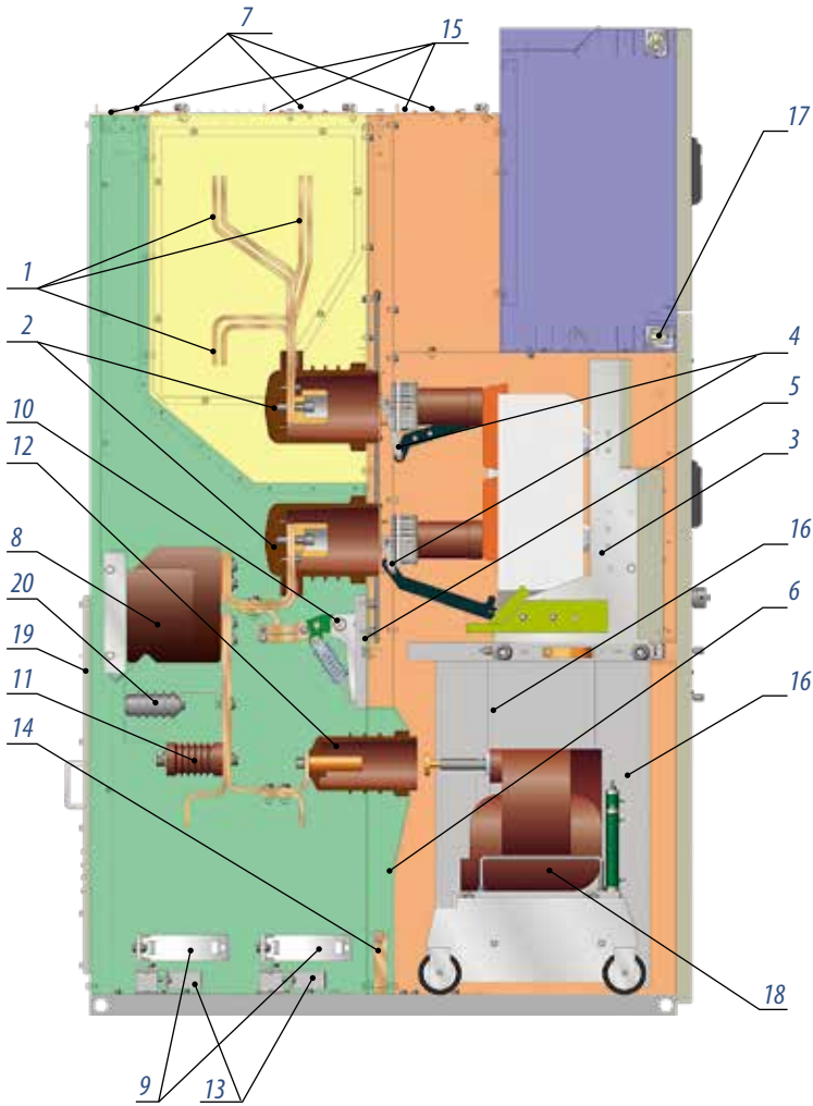
Рис. 6. Пример шкафа с силовым выключателем и ТН. Кабельный ввод снизу
