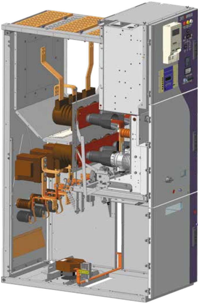
Рис. 1. КРУ «Элтима». Общий вид
