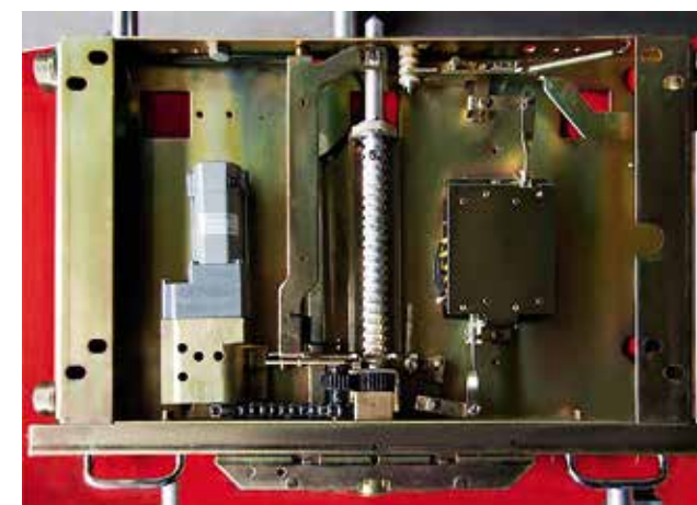
Рис. 17. Моторизированный привод КВЭ
