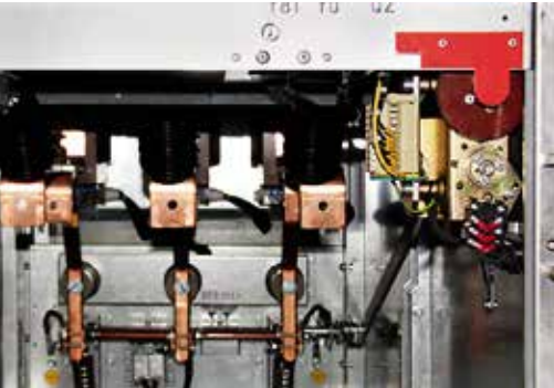
Рис. 24. Моторизированный привод заземлителя
