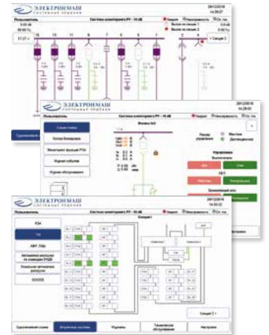
Рис. 33. Экраны системы мониторинга и управления КРУ
