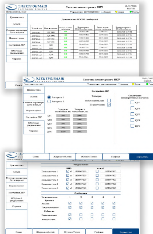
Рис. 27. Экраны системы мониторинга и управления НКУ
