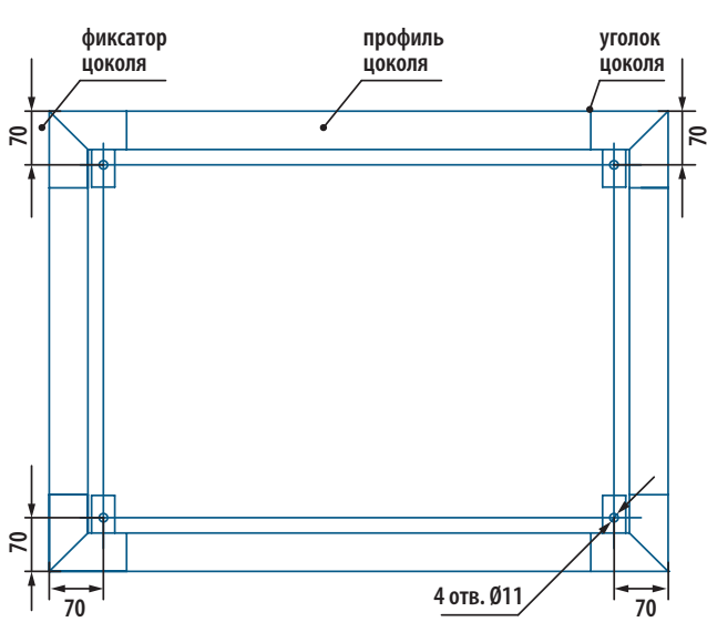
Рис. 29. Места крепления цоколя фиксаторами
