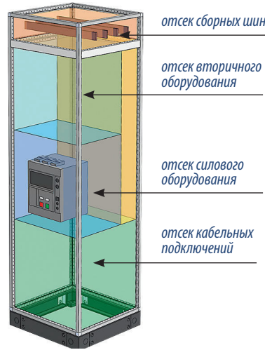
Рис. 8. Разделение шкафов ШВ и ШС на отсеки
