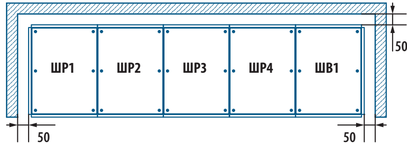
Рис. 32. Минимальные расстояния до стен помещения
