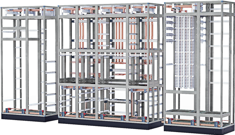
Рис. 2. Конструктив НКУ «Ассоль» (без оболочки)
