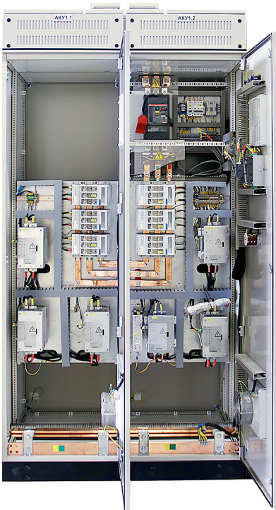
Рис. 18. Пример шкафов КРМ
