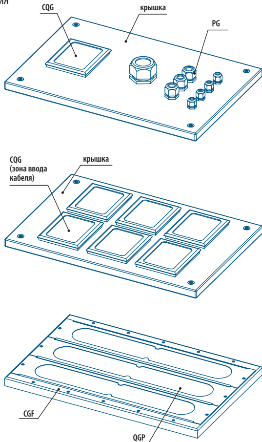
Рис. 34. Варианты прохода кабеля через сальники PG, CQG, QGP
