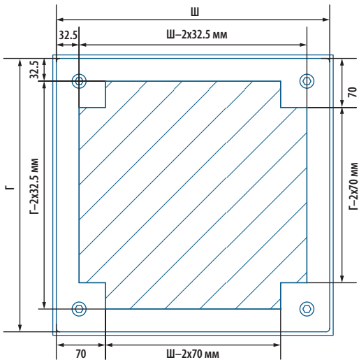
Рис. 33. Зона ввода кабелей
