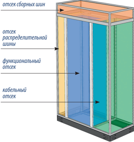
Рис. 9. Разделение шкафа ШР на отсеки
