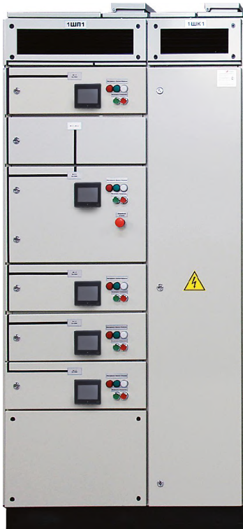
Рис. 14. Пример ШЛ с модулями фиксированного исполнения
