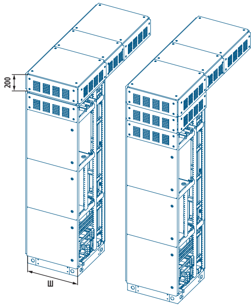
Рис. 21. Пример подключения шинного моста
