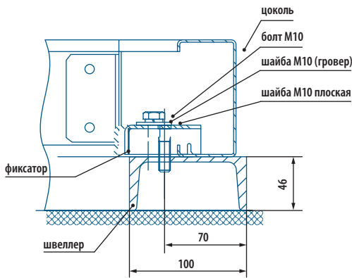
Рис. 31. Крепление цоколя к раме с помощью фиксаторов
