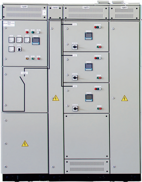
Рис. 23. Пример РУНН 0.4 кВ с обеспечением технического учета на вводах и всех отходящих линиях
