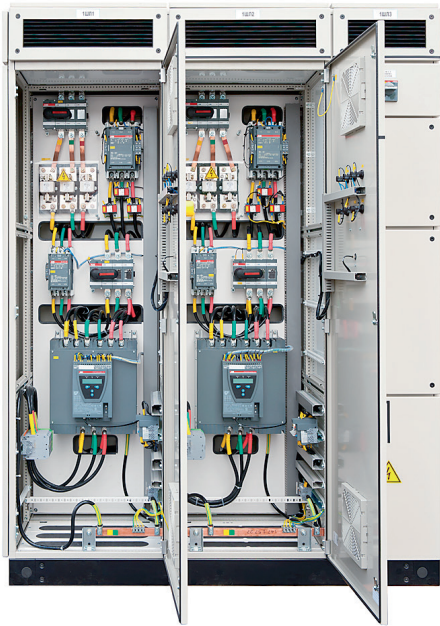
Рис. 16. Пример шкафов с фиксированным размещением УПП
