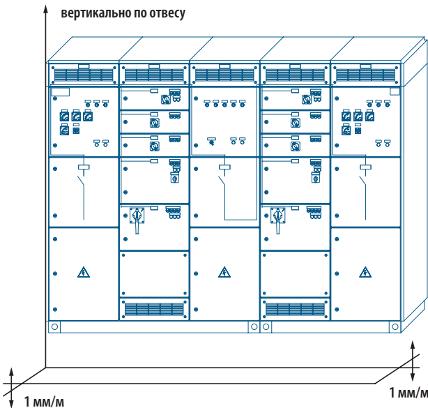
Рис. 30. Требования к фундаменту
