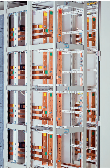
Рис. 7. Пример расположения распределительных шин
