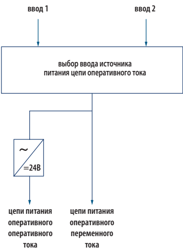
Рис. 22. Цепи оперативного тока
